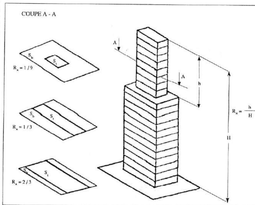
Figure 1 : Bâtiment décroché avec ses trois vues en plan.
